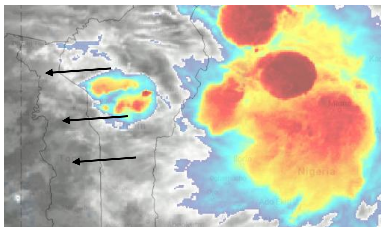
L'EVOLUTION DE L'IMAGE SATELLITAIRE DU 08/08/2026 A 04 H 45 min
